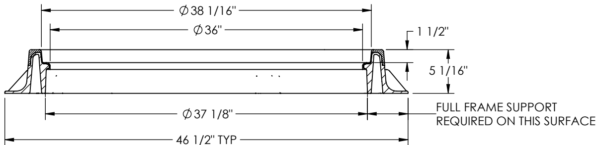
SECTION A-A
